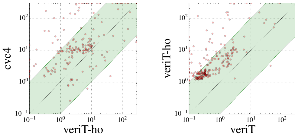
FIGURE 3.5 – Comparaisons des temps d'exécutions des solveurs cvc4 veriT et veriT-ho sur les problèmes QF_UF.
