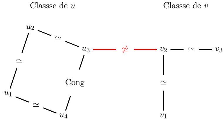
FIGURE 4.5 – Configuration de conflit si les classes u et de v doivent être fusionnées
