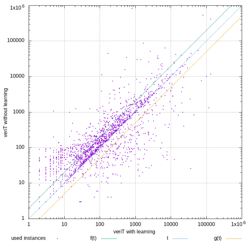
FIGURE 5.5 – Comparaison du nombre d’instances générées par les configurations veriT avec et sans apprentissage sur les benchmarks SMT-LIB UF (les 1914 benchmarks)
